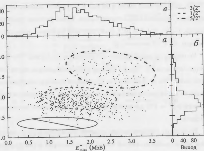
Энергия возбуждения ^{17}\text{Ne} : а Диаграмма рассеяния для энергии возбуждения измеренной методом недостающей массы ( E_{\text{miss}}^* и методом комбинированной массы ( E_{\text{comb}}^* ). Эллипсы указывают локусы вмещающие 68% событий для состояний 3/2^- , 1/2^+ (см. легенду). б Спектр комбинированной массы. в Спектр недостающей массы.
