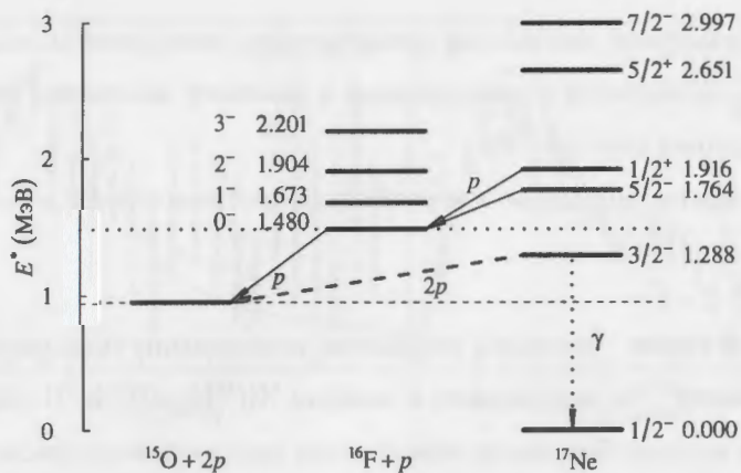
рис. 4. Схемы уровней изотопа ^{17}\text{Ne} и его подсистемы ^{16}\text{F} и схема возможных распадов для состояний ^{17}\text{Ne} .
