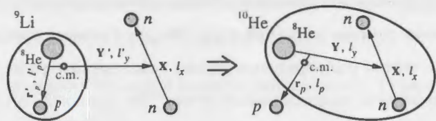
Рис. 1. Схемы координат, используемые для расчетов выбивания протона (кластера в общем случае).
