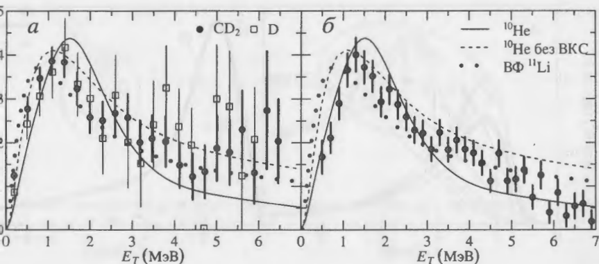
3. Сравнение расчетов спектра ^{10}\text{He} с результатами экспериментов [17] (панель а) и панель б). Сплошная черная кривая показывает сумму компонент спектра ^{10}\text{He} , представленных на Рис. 2б. Серая пунктирная кривая показывает результаты расчета спектра без учета ВКС. Серые точки показывают Фурье-Образ волновой функции ^{11}\text{Li} .
